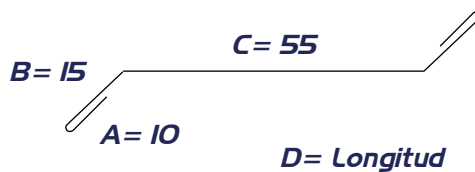
045 Luver
