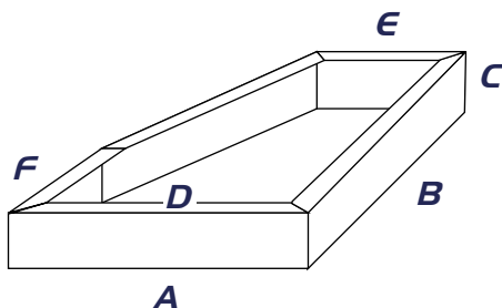
053 Charola Mensular Ceja Doble 054 Charola Dos Cejas Invertidas
