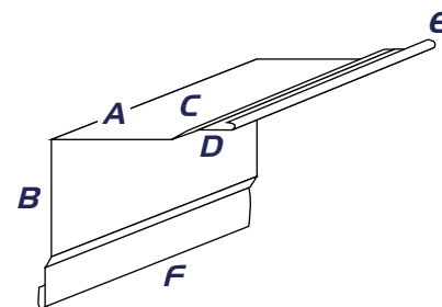
103 Perfil Int Horno
