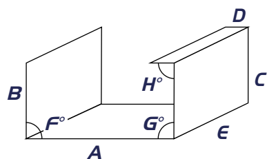
027 Canal Una Ceja Doble Interior
