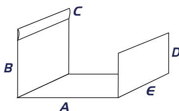
028 Canal Una Ceja Planchada
