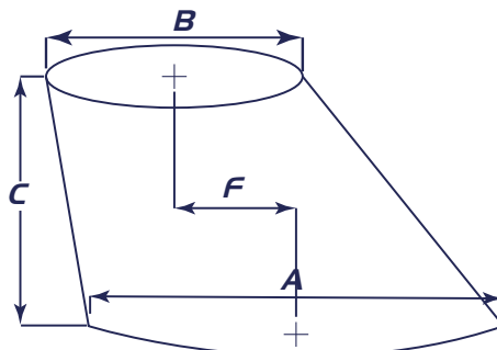
124 Reducción Excéntrica General
