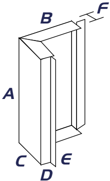
095 Perfil Esquinero T
