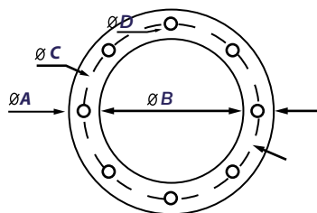
106 Brida Barrenada
