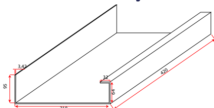
027 Canal Una Ceja Doble Ext
