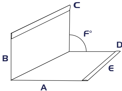
015 Ángulo 2 Lados Planchados
