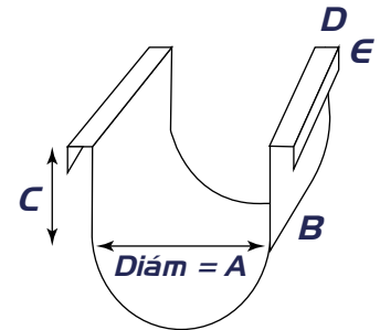
071 Artesa Ceja Doble
