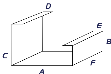
022 Canal Cejas Diferentes Doble 023 Canal Una Ceja Doble
