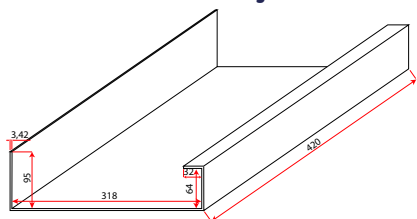
027 Canal Una Ceja Doble Int
